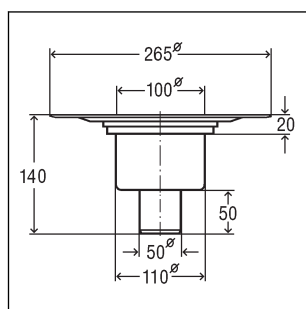
Afb. 5: Maatschets model 4926.5
