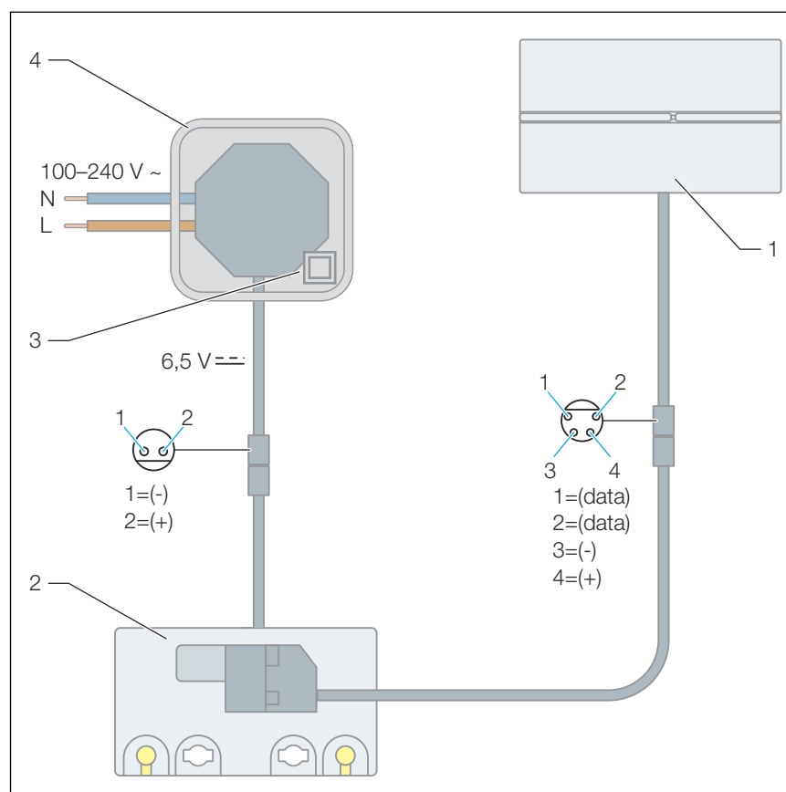
Fig. 2: Schema di collegamento, alimentatore di rete, piastra di comando per WC per Prevista
