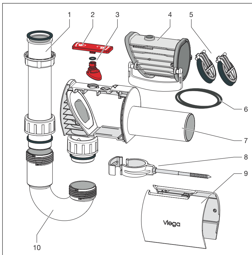
Abb. 2: Lieferumfang
