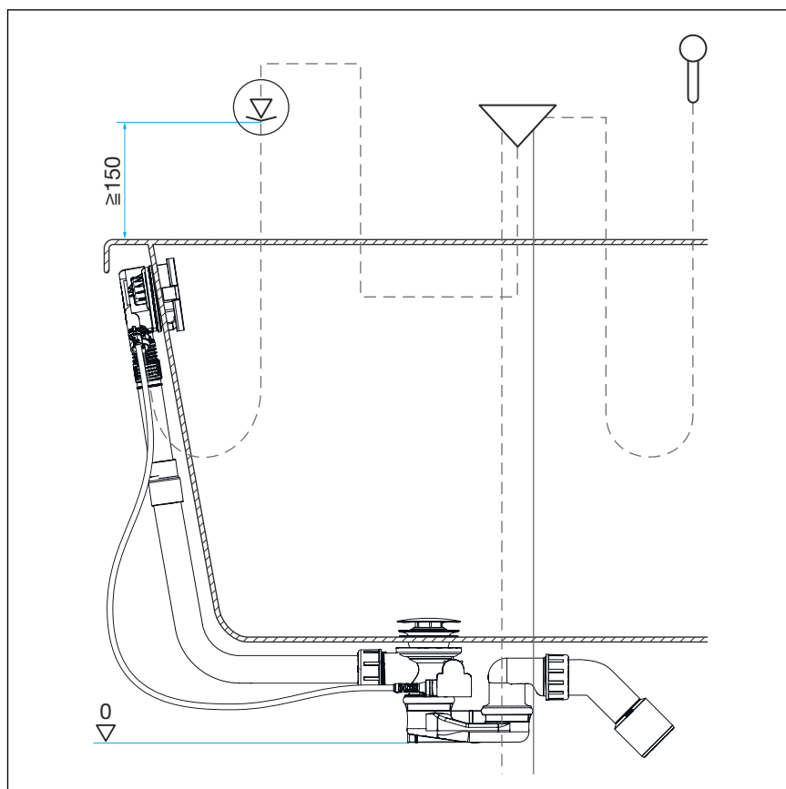
Abb. 4: Mindesteinbauhöhe 150 mm
