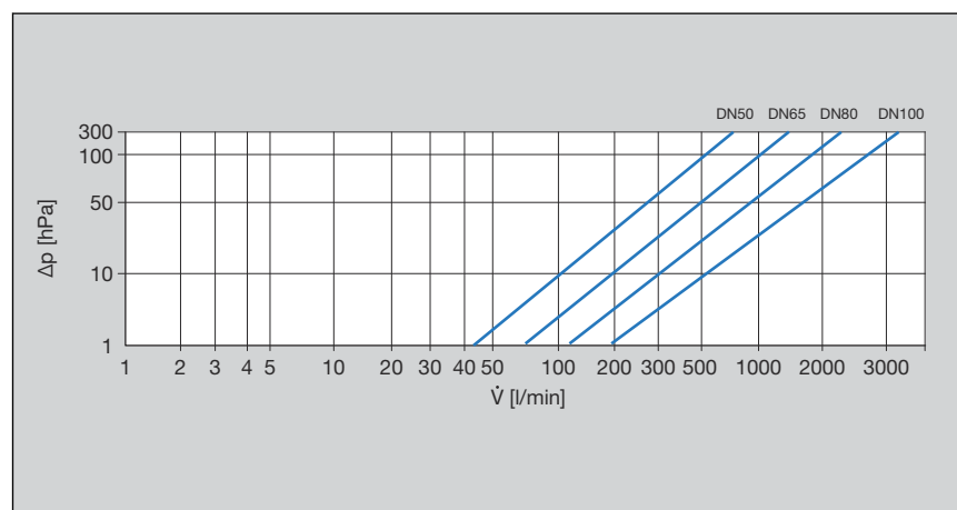
Slika 1: Dijagram učinka, pad tlaka, KRV, XL kosi nasjedni ventili, prirubnički priključak
