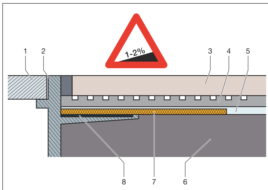
Abb. 2: Aufbauschema der Verbundabdichtung – Estrichgefälle min. 1–2 %
