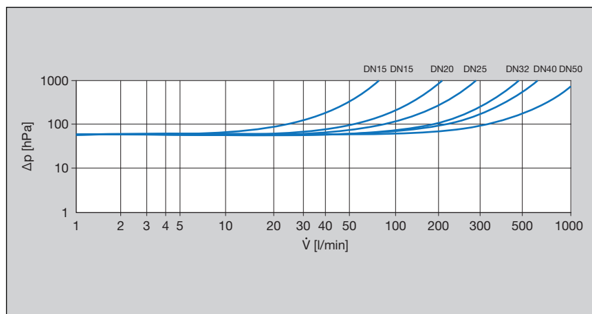
Abb. 3: Leistungsdigramm Druckverlust RV Press-/Gewindeanschluss
