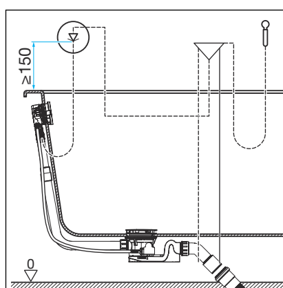
Slika 2: Shema ugradnje s prekidačem cijevi
