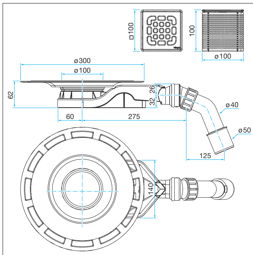
Abb. 7: Maßzeichnung Modell 4980.61
