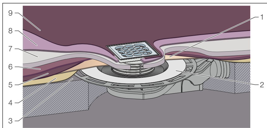
Abb. 8: Schichtaufbau der Verlaufsbeschichtung
