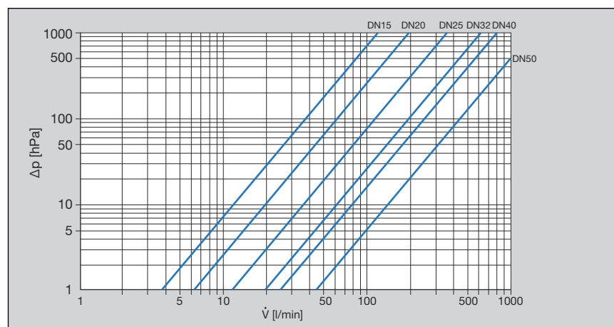
Fig. 1: Diagramma di prestazione valvole inclinate estremità a pressare femmina/filettata
