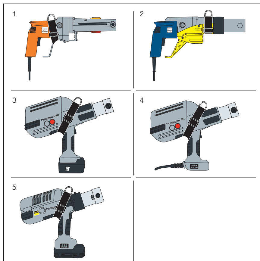
Abb. 2: Position des Spanngurts an Viega Pressmaschinen
