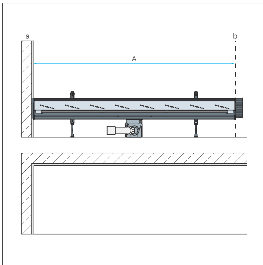
Aft. 4: Douchegoot in de hoek: gemetselde wand links, glasafscheiding rechts, afsluitkap rechts aan de buitenkant gelegen
