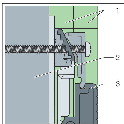
Afb. 20: Lichte constructiewand met twee gipskartonplaten, elk 12,5 mm
