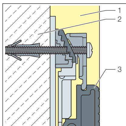
Afb. 18: Wand met 25 mm pleisterlaag
