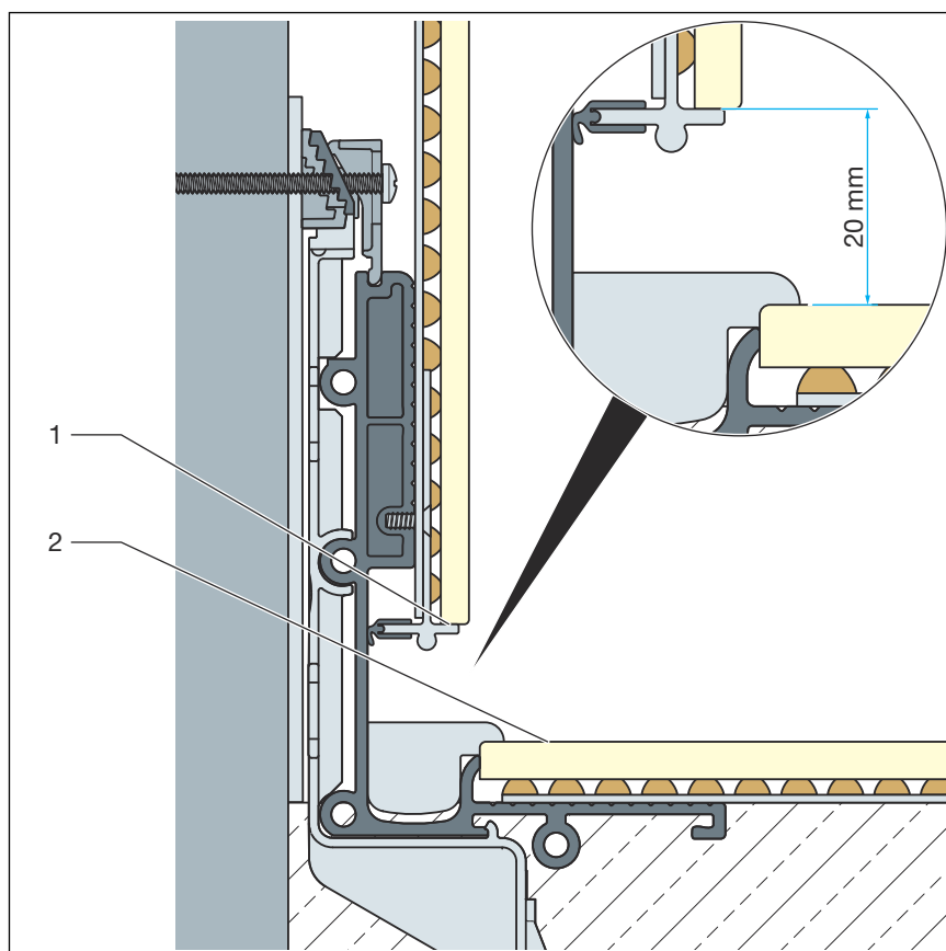
Afb. 22: Afsluitprofiel in ingebouwde toestand, wand- en vloertegels gelegd
