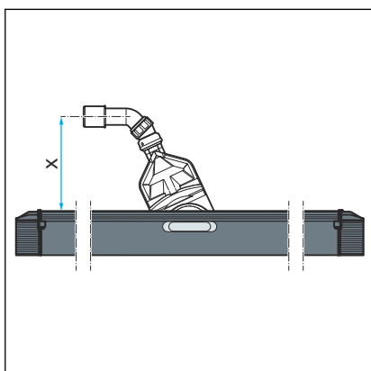
Afb. 11: Model 4966.18 (renovatiemodel)
