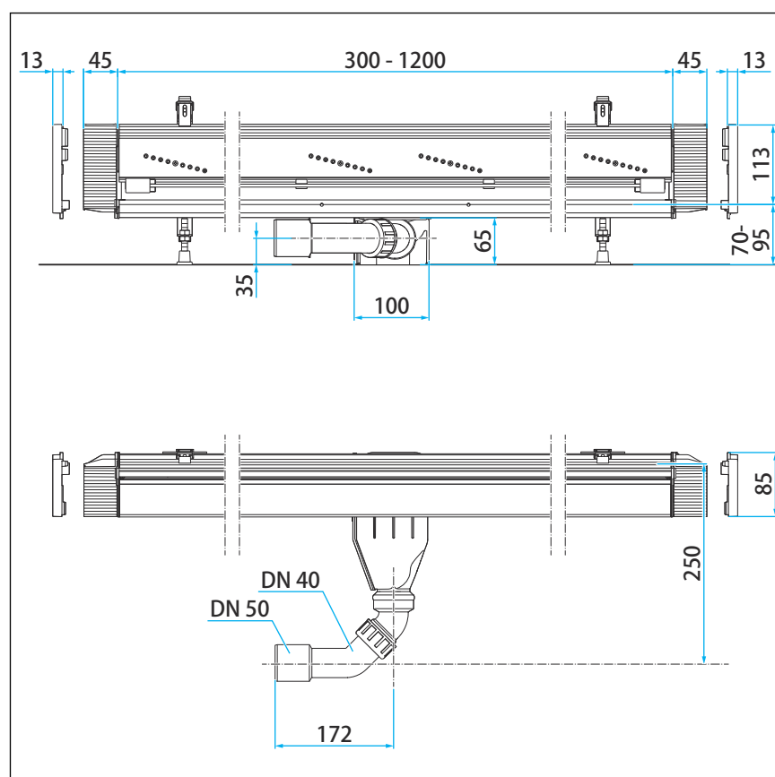
Slika 17: Dimenzije osnovnog modela osnovnog kućišta
