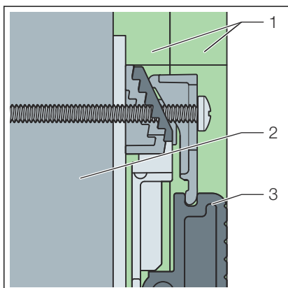
Slika 20: Montažni zid s dvije gips-kartonske ploče od po 12,5 mm
