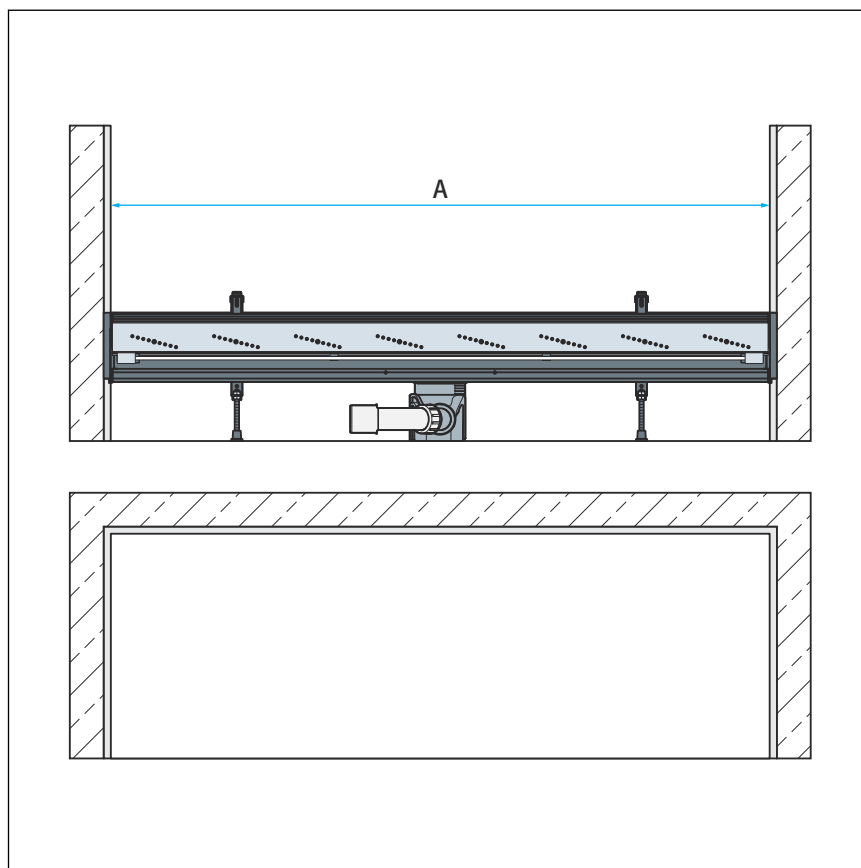
Slika 2: Tuš kanalica u niši: ozidani zid lijevo i desno
