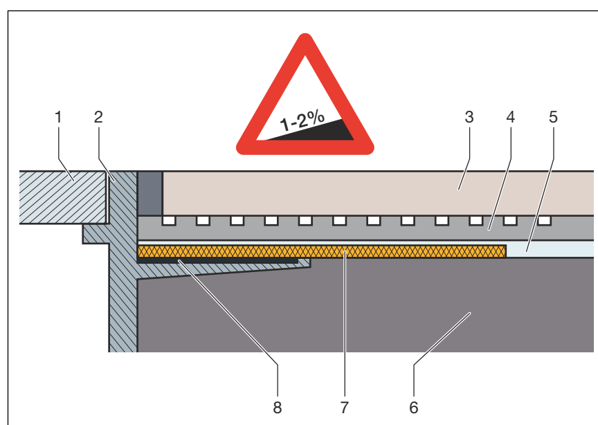
Slika 14: Shema konstrukcije hidroizolacijskog premaza – min. nagib estriha 1-2 %
