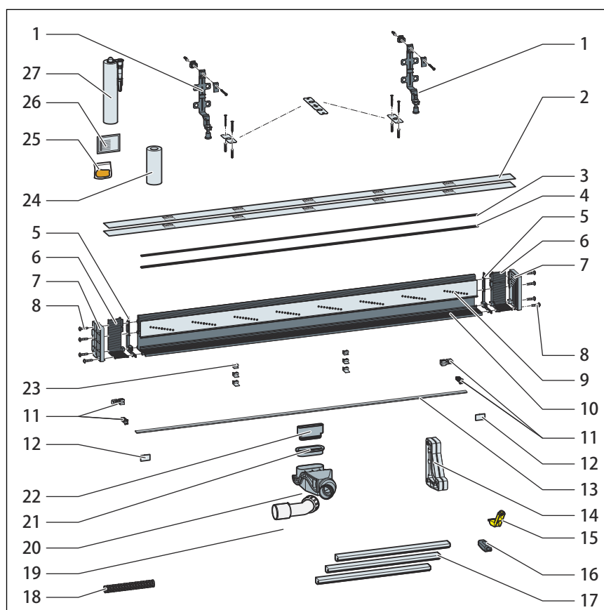
Fig. 12: Composants et matériel fourni
