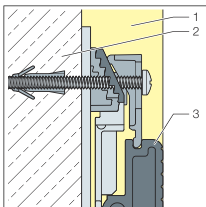
Fig. 18: Mur avec une couche d'enduit de 25 mm
