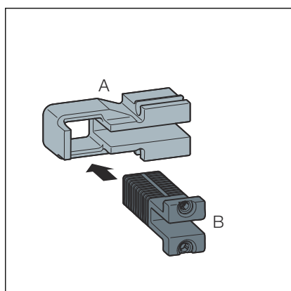
Fig. 23: Paire de supports pour élément de finition
