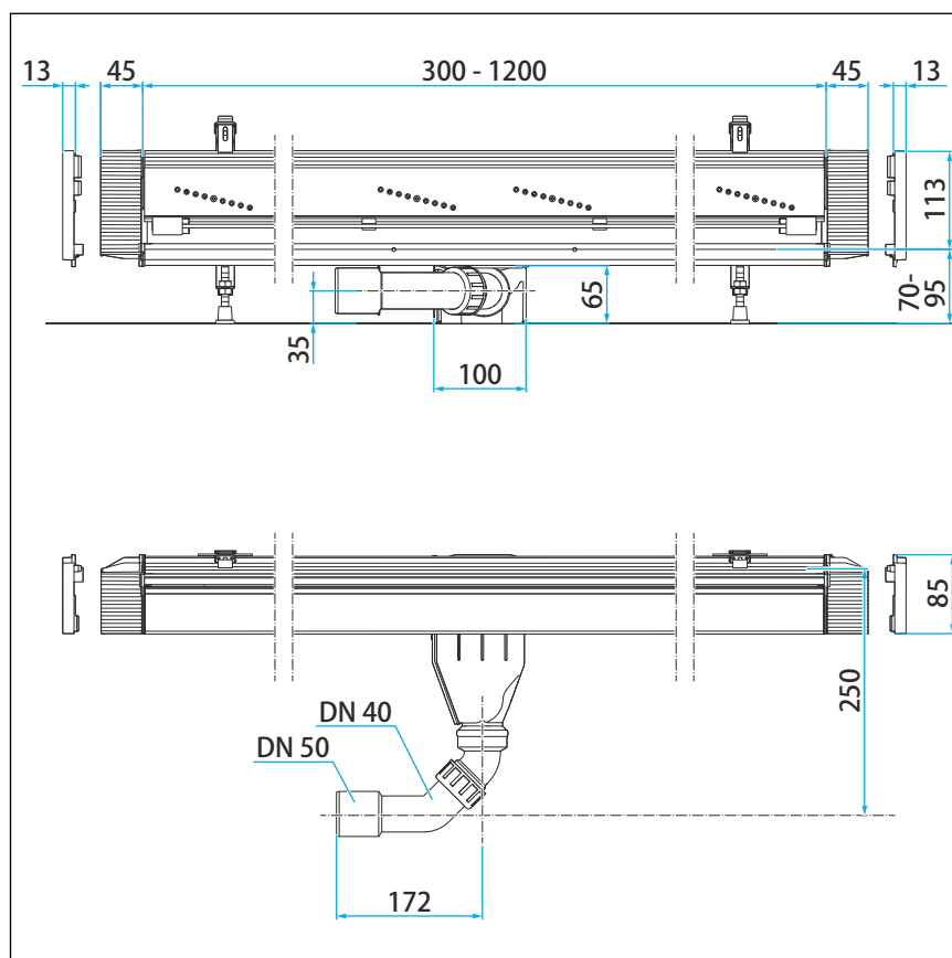
Fig. 17: Dimensions unité de base modèle de base
