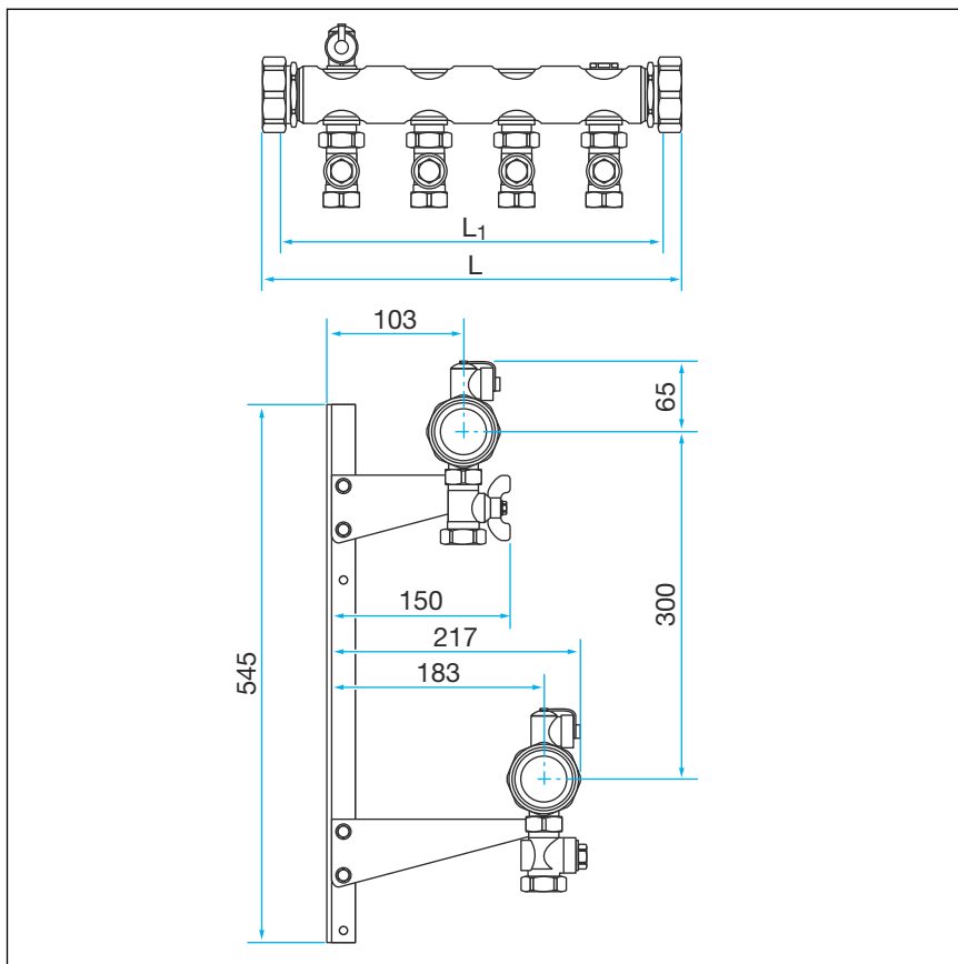
Abb. 3: Maßzeichnung 2
