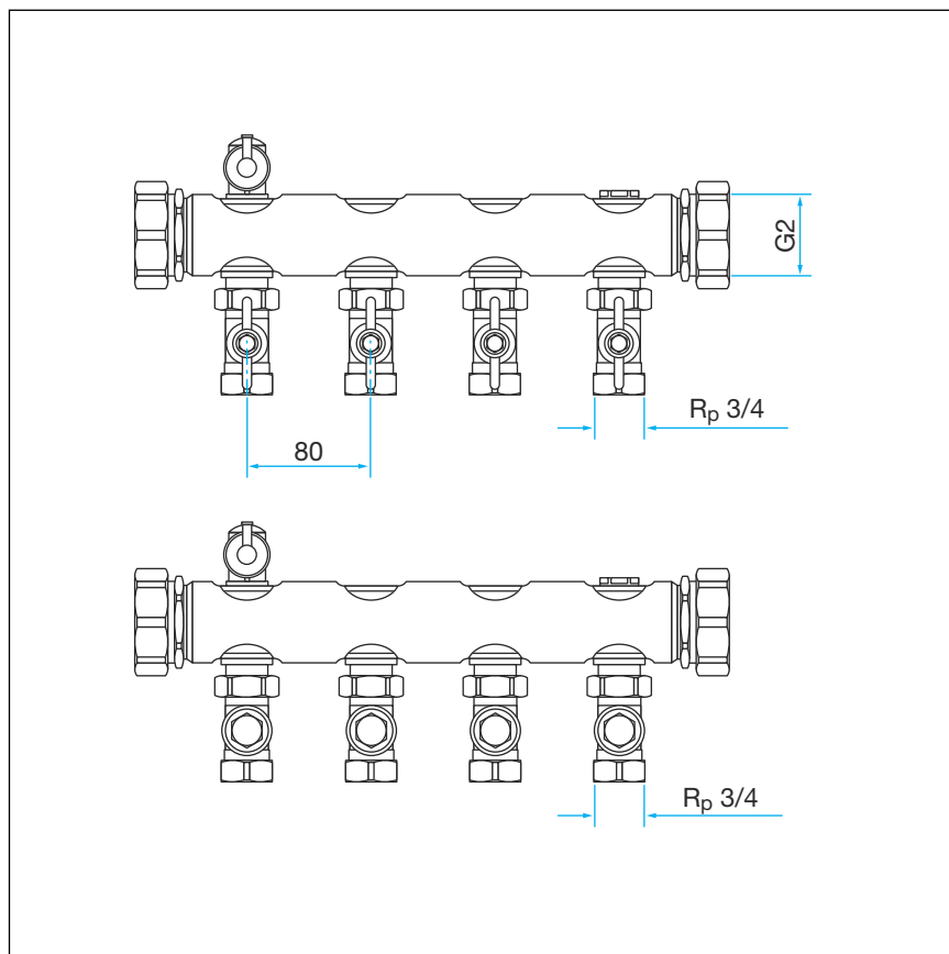
Abb. 2: Maßzeichnung 1
