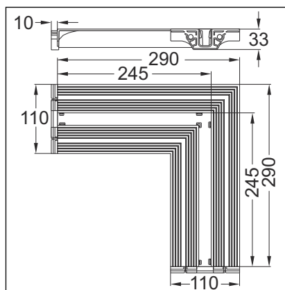
Afb. 6: Afmetingen
