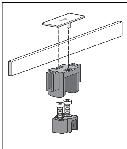
4. ábra: Járóléckészlet
