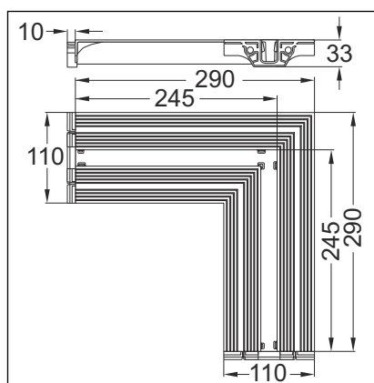
Slika 6: Dimenzije
