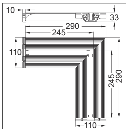
Fig. 6: Dimensions pièce de raccordement 90°
