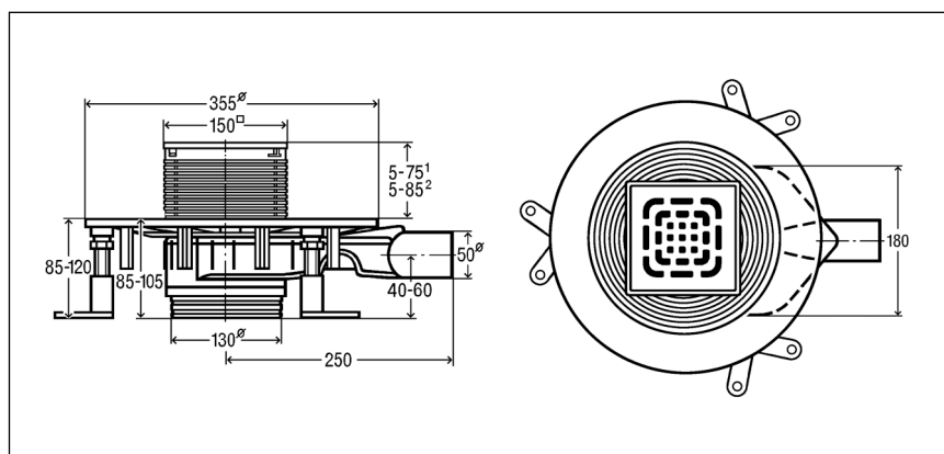
Obr. 7: rozmerový výkres modelu 4914.21
