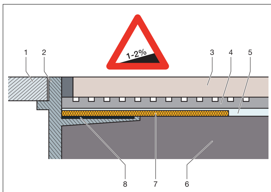
Obr. 5: schéma štruktúry spojeného utesnenia – sklon poteru min. 1–2%
