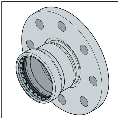
Fig. 7: Flangia fissa
