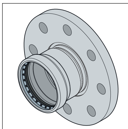
Fig. 7: Brida fija
