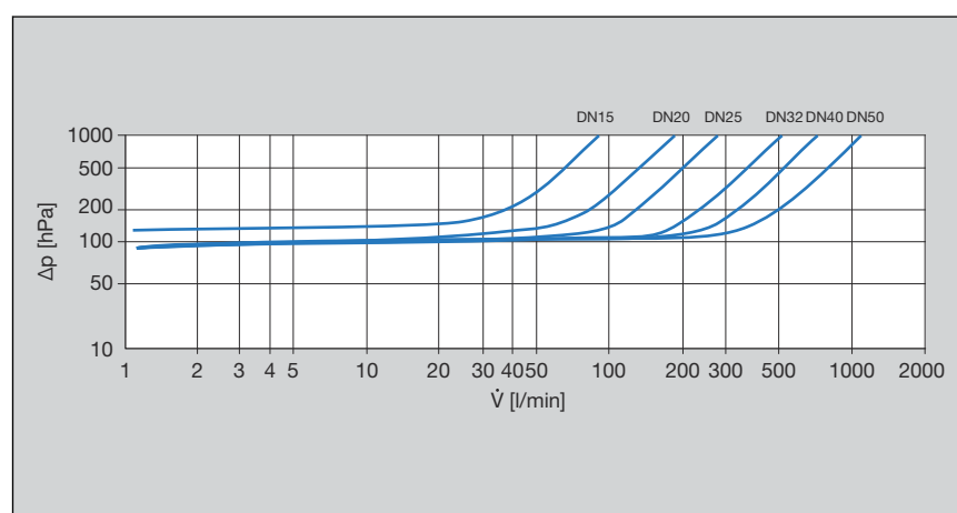
Abb. 3: Leistungsdiagramm Druckverlust KRV Press-/Gewindeanschluss
