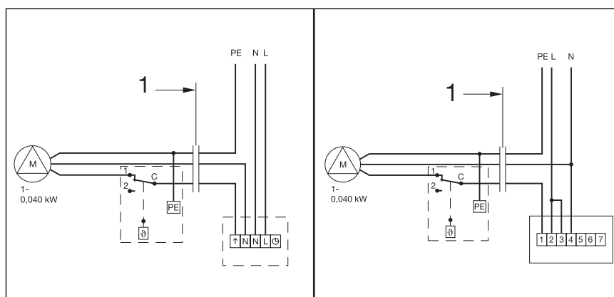
Fig. 4: Schema di collegamento per un termostato ambiente Viega 230 V (sinistra), termostato con orologio 230 V (destra)
