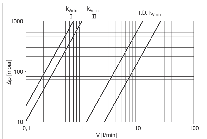
Abb. 2: Diagramm Betriebsarten / Druckverluste
