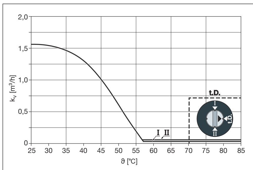
Abb. 1: Diagramm Mindestdurchfluss / Temperatur
