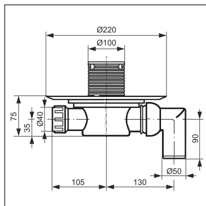
Bild 7: Ritning för modell 4935.3
