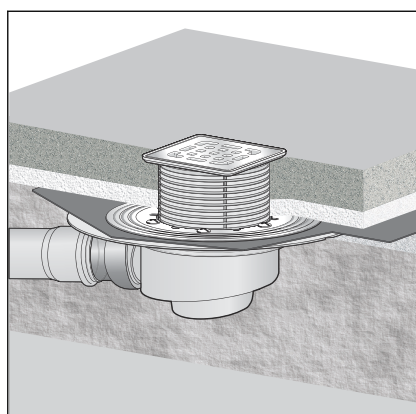
Bild 1: Allmänt monteringsexempel – takurspärning
