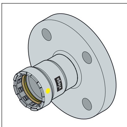
Afb. 10: Vaste flens
