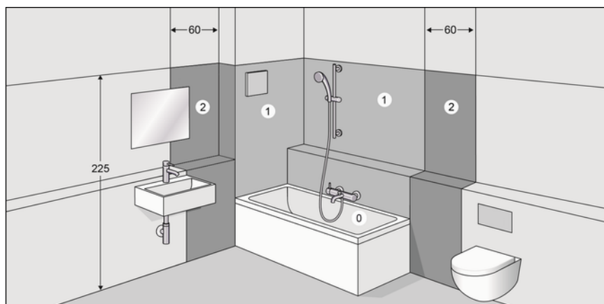
Afb. 10: Veiligheidszones
