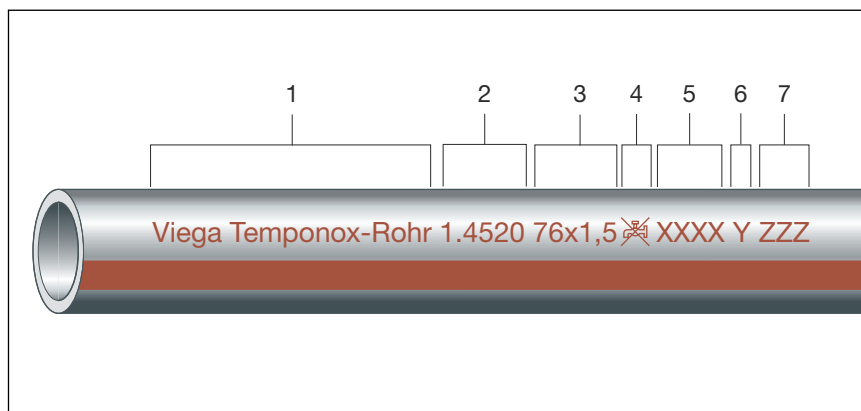
Abb. 6: Temponox-Rohr 1.4520
