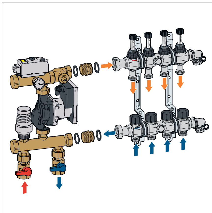
Abb. 5: Montagebeispiel mit Regelstation
