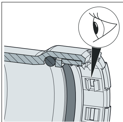
Abb. 10: Schneidring
