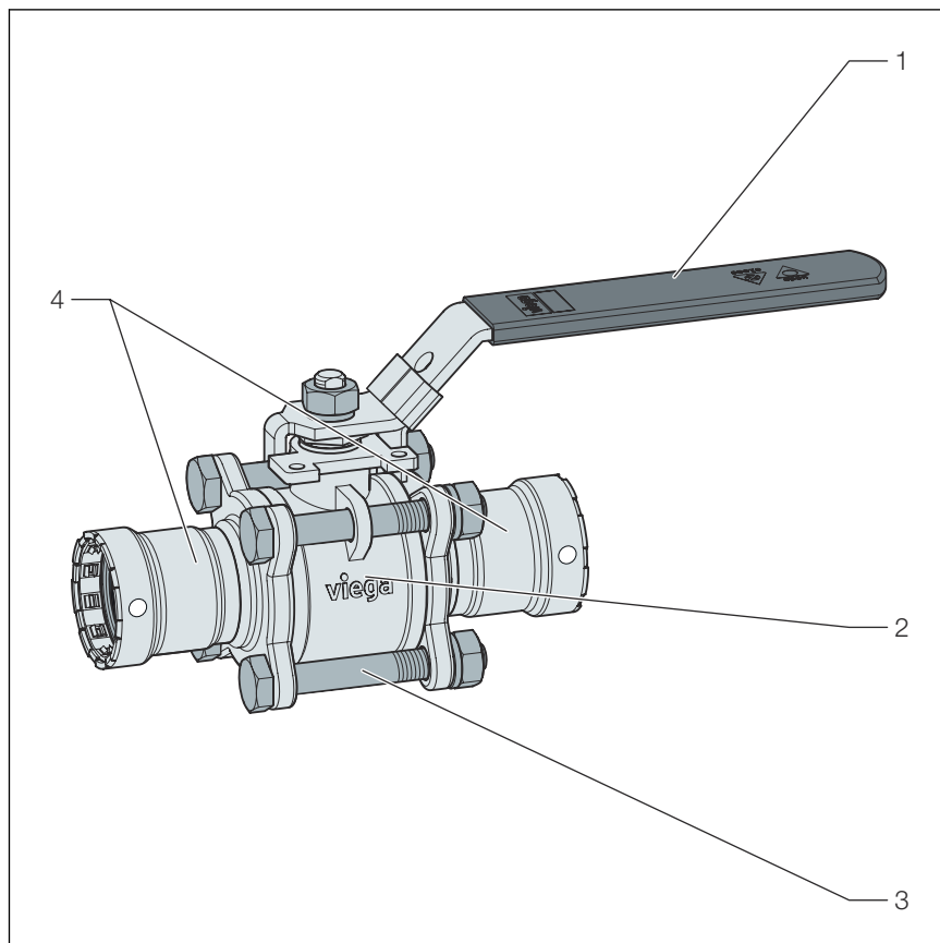
Abb. 2: dreiteiliger Kugelhahn
