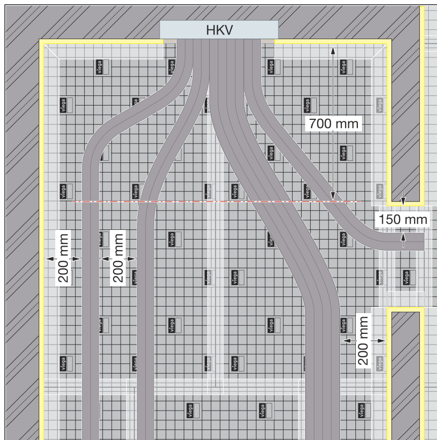
Abb. 2: Mindestabstände und Biegeradien
