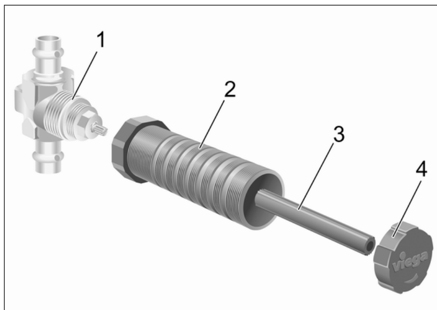
Fig. 1: Struttura di una valvola a sede dritta in base all'esempio del modello 2235
