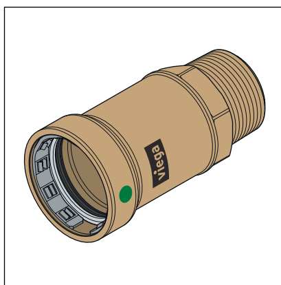
Slika 1: Megapress prijelazni komad na R-navoj (model 4211.4)
