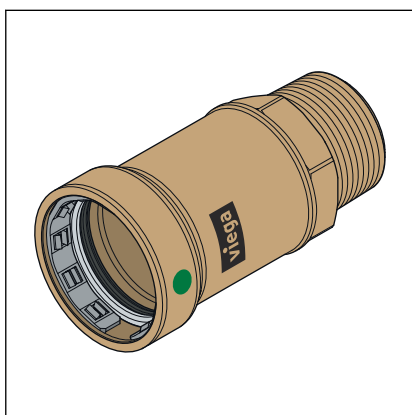
Slika 2: Megapress prijelazni komad (model 4211.4)
