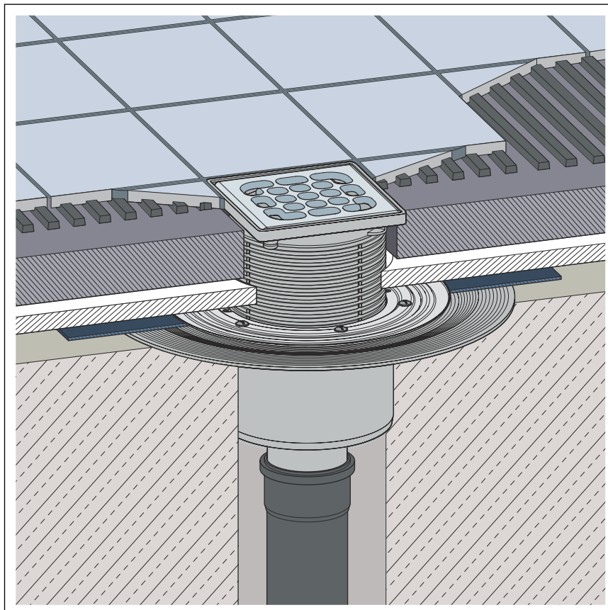
Abb. 4: Schema einer konventionellen Abdichtung
