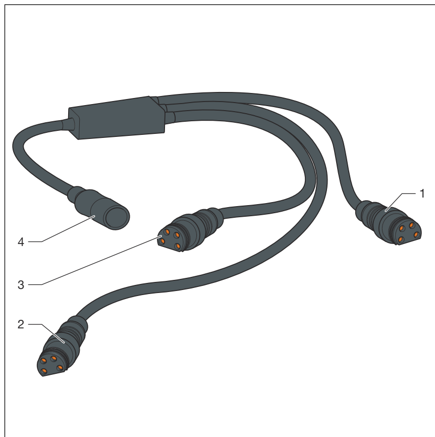
Fig. 1: Cavo adattatore per prolunga
