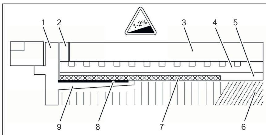
Abb. 2: Aufbauschema der Verbundabdichtung – Estrichgefälle min. 1–2 %
