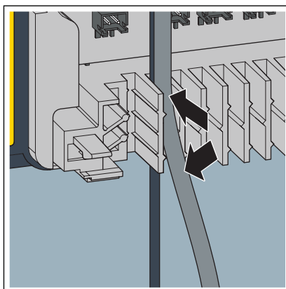
Zugentlastung mit zwei Anschlusskabeln an der Gehäuseunterseite (Temperatursensor und Stellantrieb).
