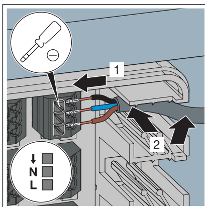
Zugentlastung an der rechten Gehäuseseite.
