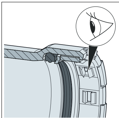
Fig. 10: ghiera dentata
