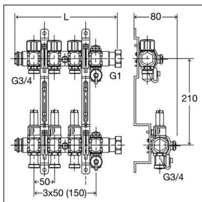
Afb. 2: Maattekening
