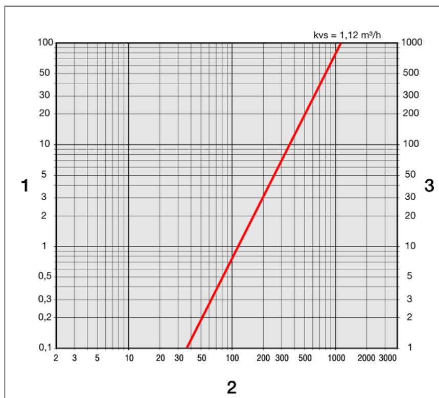
Afb. 7: Drukverlies voor debietwijzer 0–5 l/min (in de aanvoerleiding)
