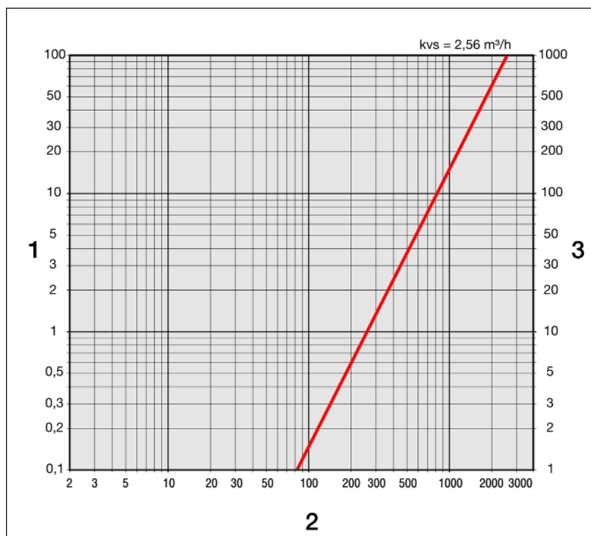
Afb. 6: Drukverlies voor thermostaatventiel (in retour)
