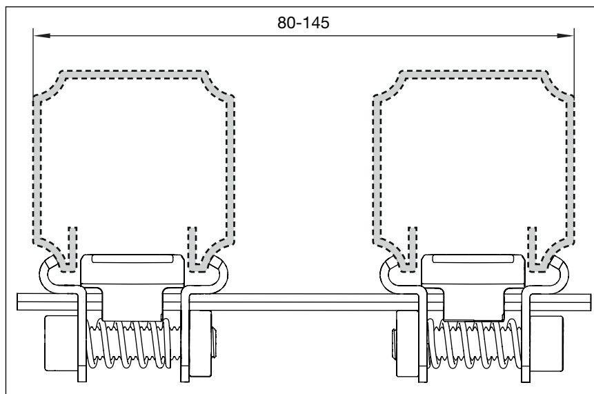
2. ábra: Méretraajz
