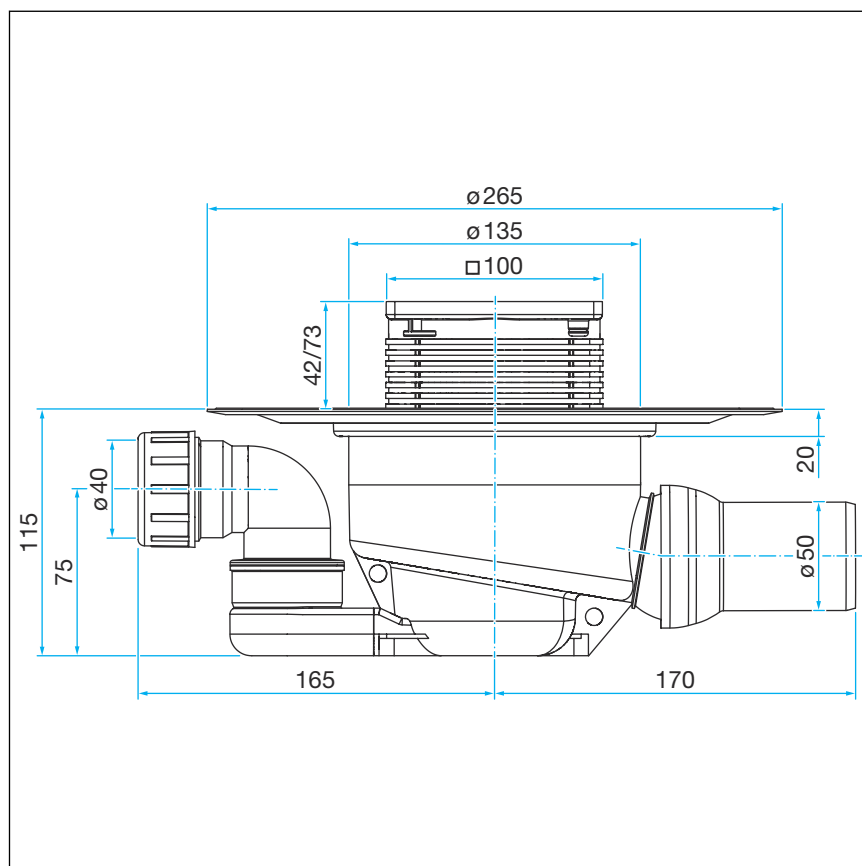
Fig. 7: Schéma coté modèle 4921.6
