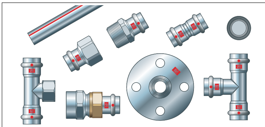
Fig. 2: Selezione gamma Prestabo
