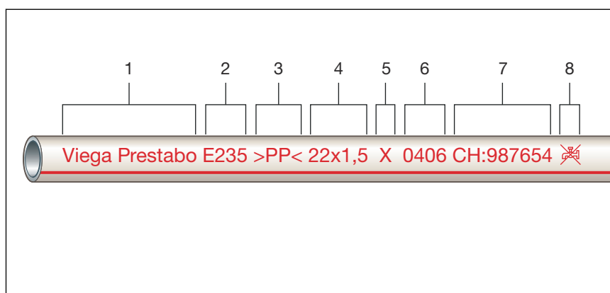
Fig. 7: Tubo rivestito in PP
