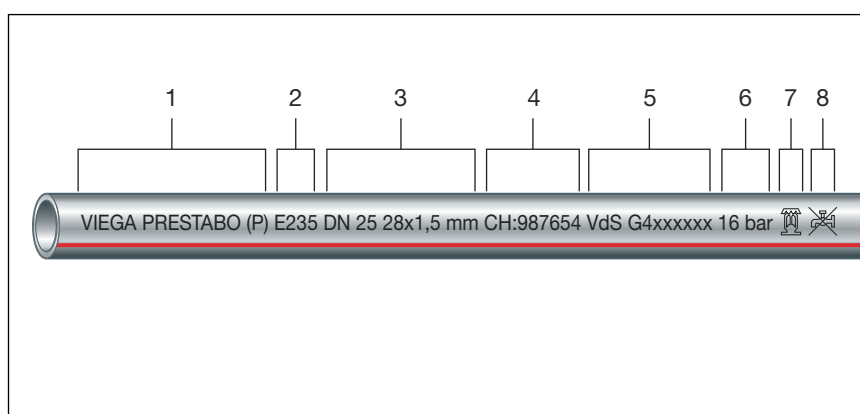
Fig. 8: Tubo zincato sendzimir internamente e esternamente
