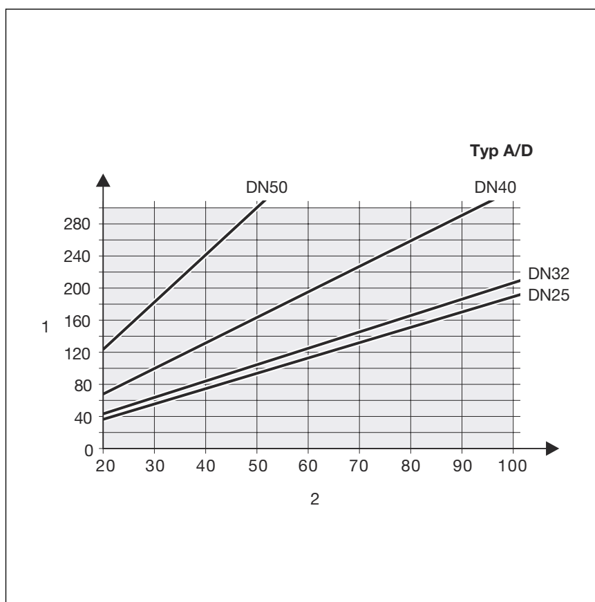
5. ábra: Irányadó értékek megfúróidomhoz és főelzáróhoz, \zeta=10 alaki ellenállástényezőhöz
