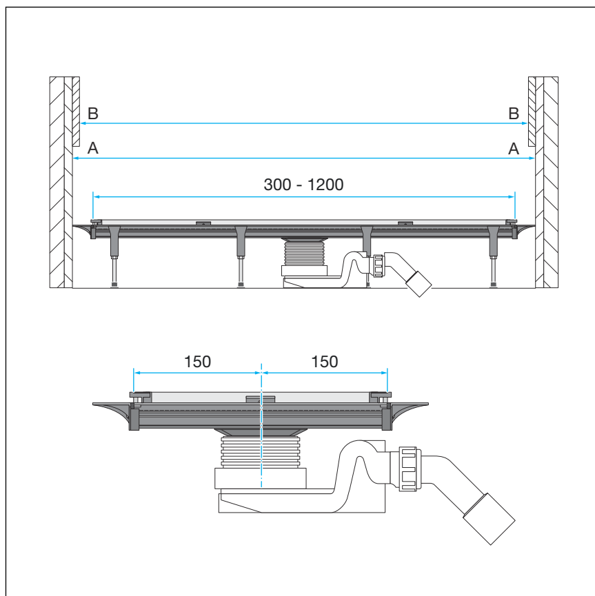
Slika 18: Dimenzije niše
