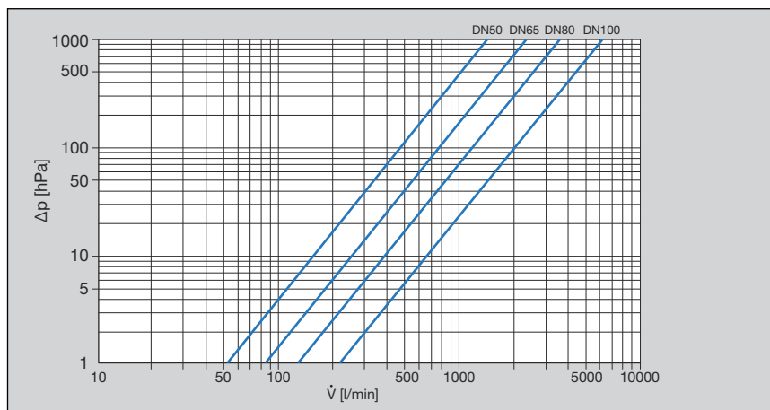
Slika 1: Dijagram učinka, pad tlaka, XL kosi nasjedni ventili, prirubnički priključak
