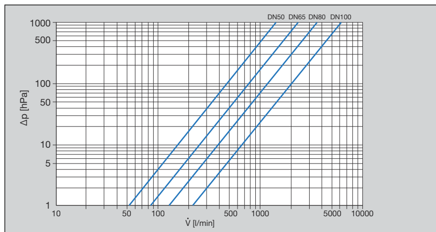
Afb. 1: Vermogensdiagram drukverlies XL schuine klepafsluiters flensaansluiting
