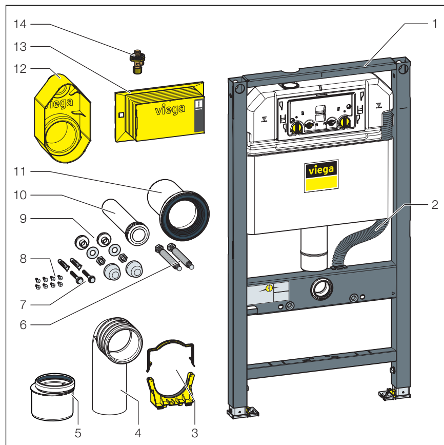
Obr. 1: Konštrukčné diely
