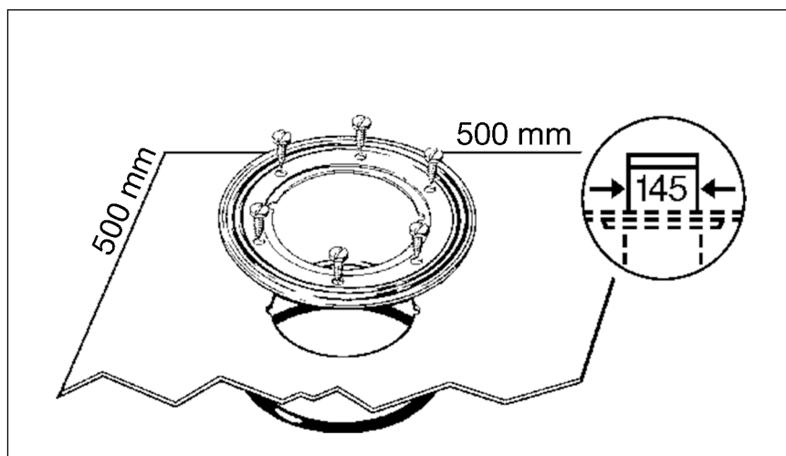
Obr. 2: Rozmery
