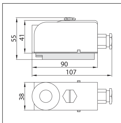
Abb. 1: Produktmaße
